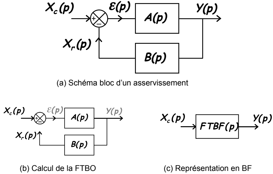
Fig. III.2 – Représentation sous forme de schéma bloc d'un asservissement.
