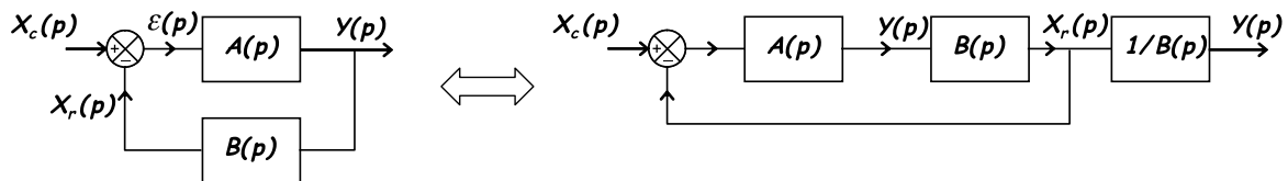
Fig. III.4 – Structure équivalente à un retour unitaire.
