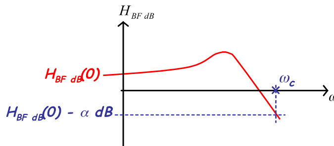
Fig. III.8 – Bande passante à -\alpha\ dB de la BF.
