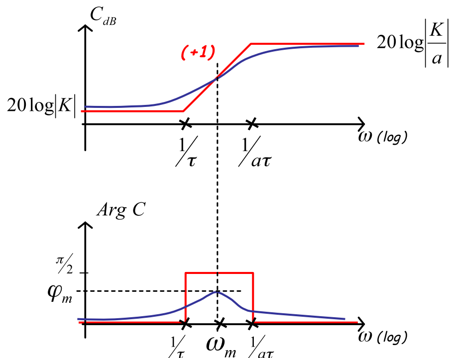
Fig. V.6 – Correcteur à avance de phase (diagramme de Bode).
