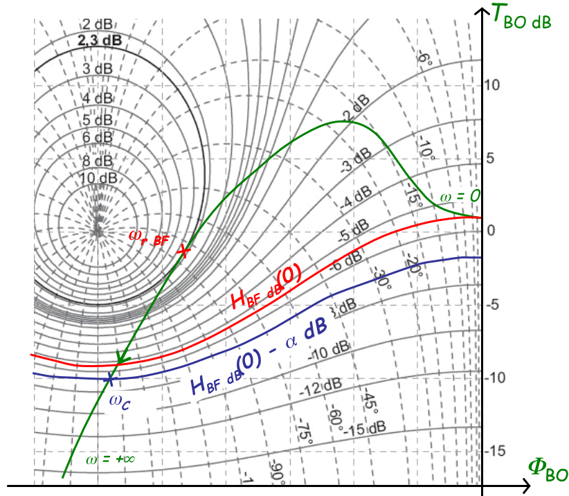
Fig. III.9 – Détermination de la bande passante à -\alpha\text{ dB} en BF.
