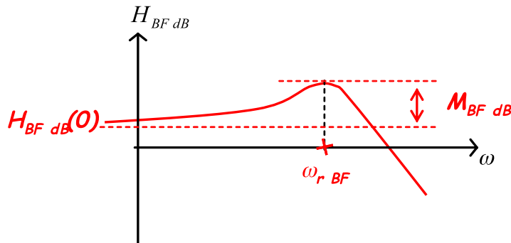
Fig. III.7 – Module en dB de la FTBF.
